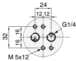
Деталь X ADA/ASR 0020U-1750U
