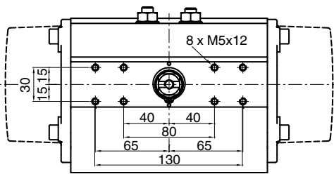
Деталь X ADA/ASR 0020U-1750U
